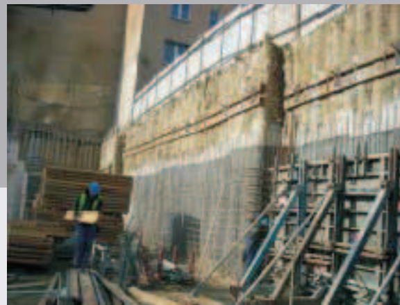
Zabezpieczenie głębokiego wykopu Filharmonia, Kielce
