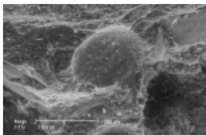
Fot. 3. Widok ogólny i skład pierwiastkowy (SEM/EDS) mikrostruktury betonu z udziałem mikrosfer w spoiwie, po 28 dniach przechowywania w środowisku wody [Fot. E. Haustein]
