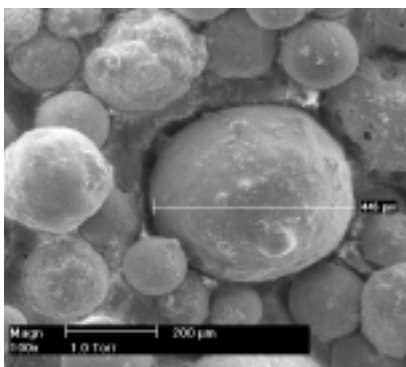
Fot. 1. Widok ogólny struktury ziaren mikrosfer. Materiał badawczy: elektrownia „Dolna Odra”, powiększenie 100x [Fot. E. Haustein]
