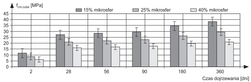
Wpływ udziału 15%, 25%, 40% mikrosfer na średnią wytrzymałość (f cm,cube ) w funkcji czasu dojrzewania betonu, w/s = 0,52
