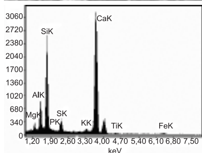
Fot. 3. Widok ogólny i skład pierwiastkowy (SEM/EDS) mikrostruktury betonu z udziałem mikrosfer w spoiwie, po 28 dniach przechowywania w środowisku wody [Fot. E. Haustein]
