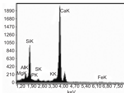
Fot. 4. Widok ogólny i skład pierwiastkowy (SEM/EDS) mikrostruktury betonu z udziałem mikrosfer w spoiwie, po 360 dniach przechowywania w środowisku wody [Fot. E. Haustein]
