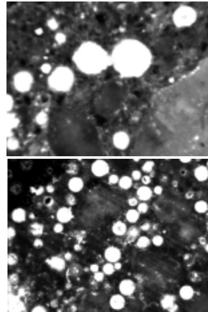
Fot. 2. Ogólny widok rozmieszczenia porów powietrznych (kolor biały, kształt kulisty) w mikrostrukturze betonu z udziałem 15% oraz 40% mikrosfer w spoiwie, po 28 dniach dojrzewania, w/s = 0,52 [Fot. E. Haustein]
