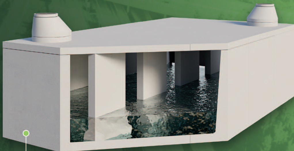
ZBIORNIKI SEGMENTOWE TYPU „U”
