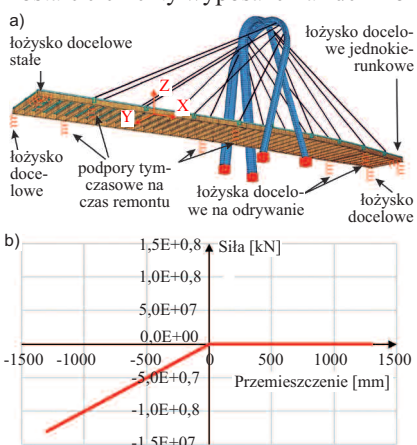
Rys. 4. Wizualizacja modelu numerycznego z opisem warunków brzegowych (a); prawo materiałowe jednostronnych podpór sprężystych (b)
