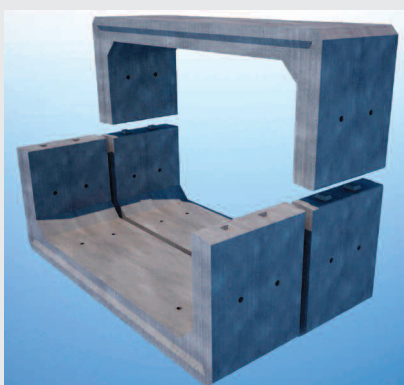
Przepusty drogowe i kolejowe z elementów prefabrykowanych
