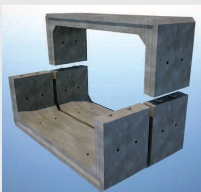
Elementy prefabrykowane do wykonywania przepustów drogowych i kolejowych
