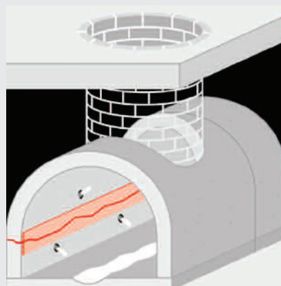
Schemat zastosowania szpachlówki epoksydowej WEBAC 4520
