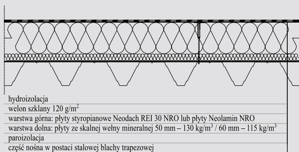
Przekrój dachu w systemie Neuroof Fireproof REI 30 NRO
