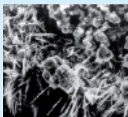
Początek krystalizacji po aplikacji XYPEX-u
