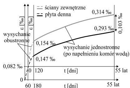
Rys. 2. Rozwój skurczu betonu w elementach zbiornika Fig. 2. Concrete shrinkage development in the tank elements
