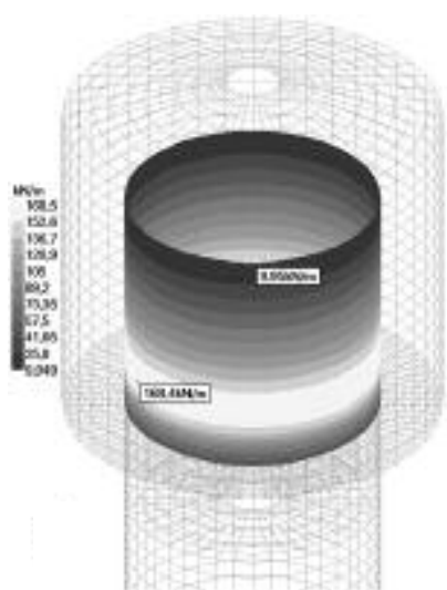
Rys. 3. Rozkład sił obwodowych w ścianach od obciążeń zewnętrznych Fig. 3. Distribution of peripheral forces in walls from external loads
