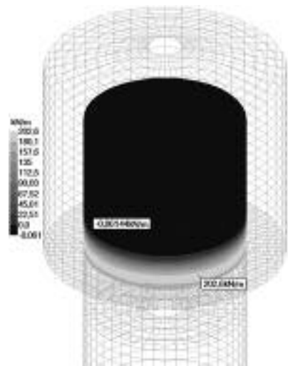
Rys. 4. Rozkład sił obwodowych w ścianach od całkowitego odkształcenia skurczowego betonu Fig. 4. Distribution of peripheral forces in walls from total shrinkage deformation of concrete
