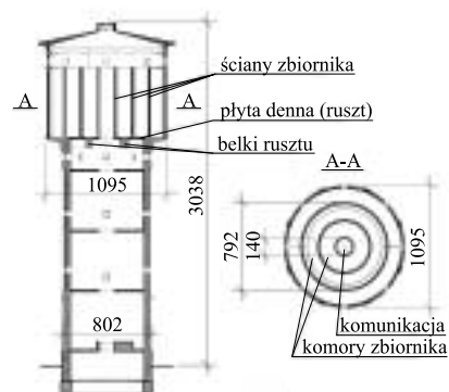
Rys. 1. Przekrój pionowy i poziomy wieży Fig. 1. Vertical and horizontal cross-section of the tower
