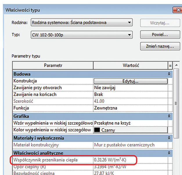
Rys. 4. Przykład obliczania współczynnika przenikania ciepła przegrody
